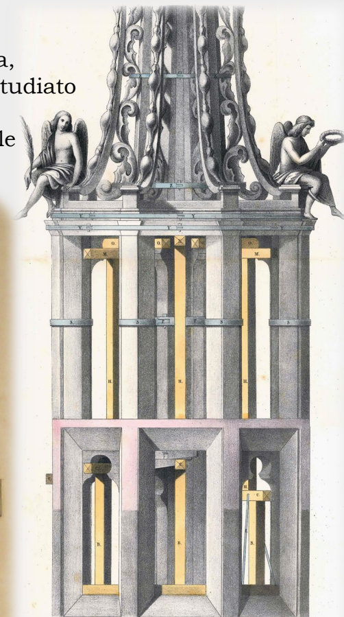
A. Nava. Progetto di consolidamento della guglia maggiore del Duomo di Milano
